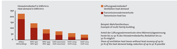
Energetischer Anteil der Lüftung am Wärmebedarf Energy share of ventilation in heat demand
